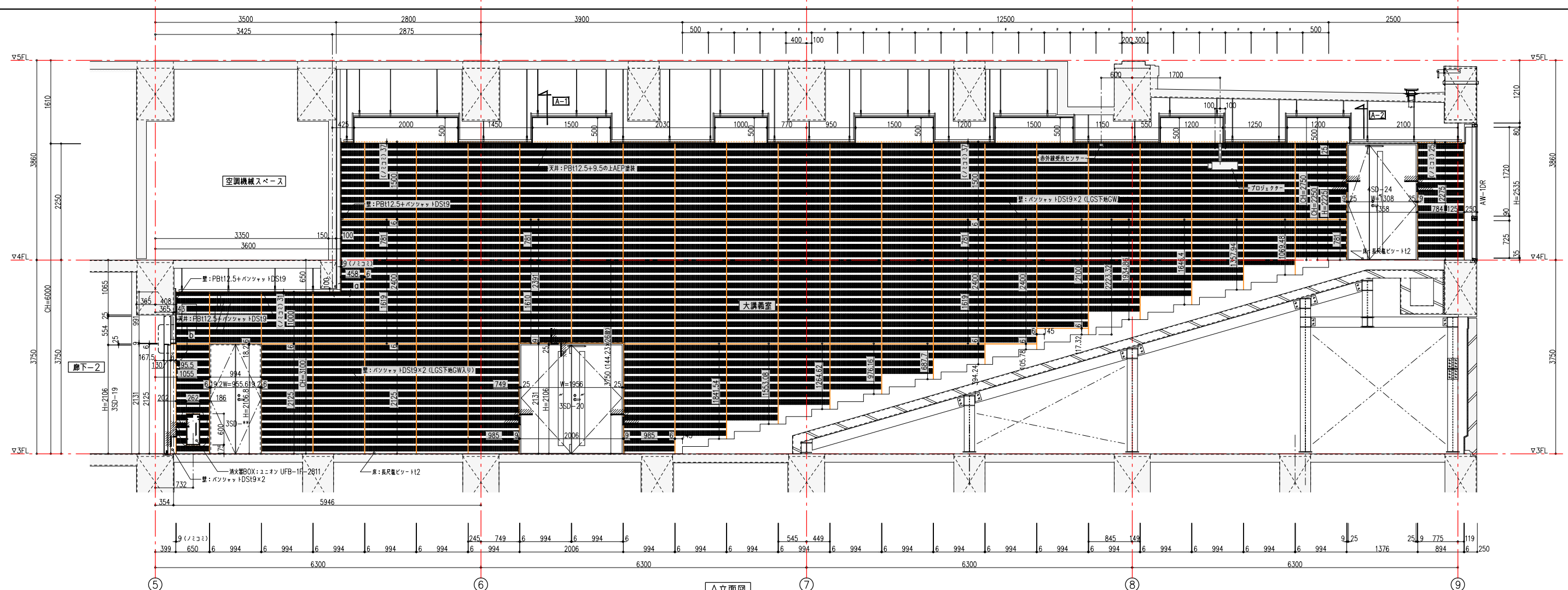
A立面図
