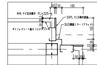
コーナー部 詳細
