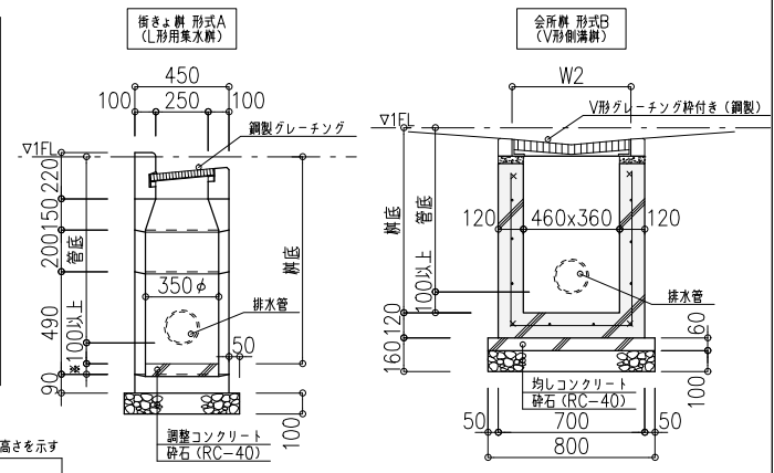
外構詳細図 S=1:20 (A1)
