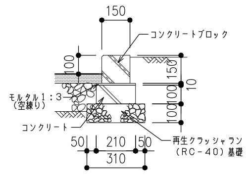
地先境界ブロックA
