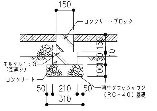
地先境界ブロックB
