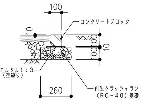
地先境界ブロックC
